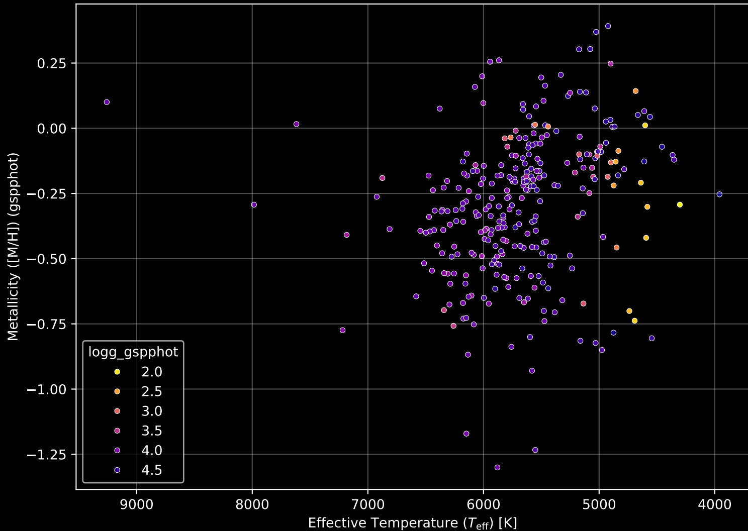
GALAH DR4 Field: [999] Stellar Population Parameters (n= 297)
