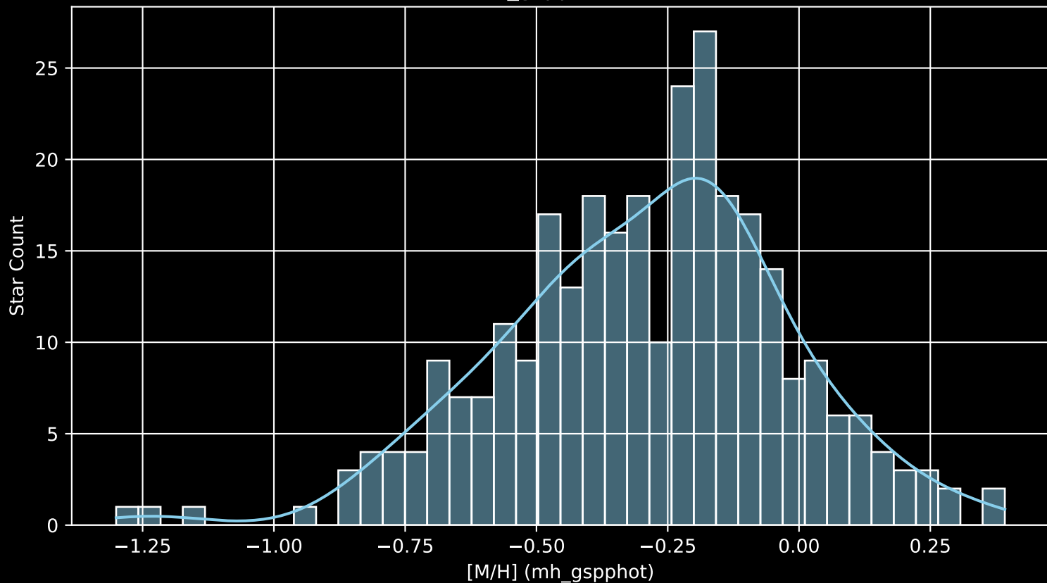
GALAH DR4 Field: [999] [M/H] (mh_gspphot) (n= 297)
