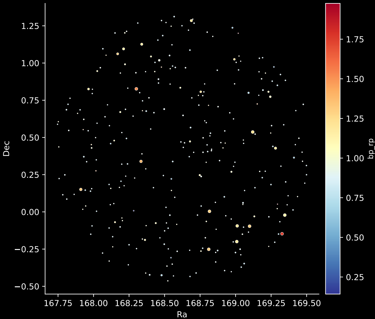
GALAH DR4 Field: [999] Stars: 297
